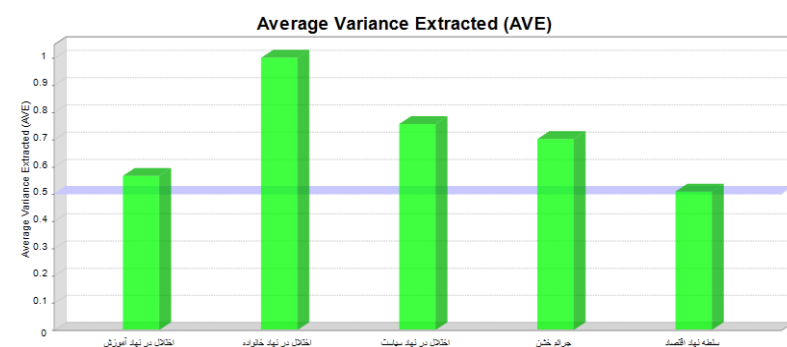
نمودار ۲: روایی همگرایی مدل
